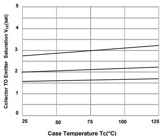
Fig. 4 V_{CE(SAT)} vs. T_C
