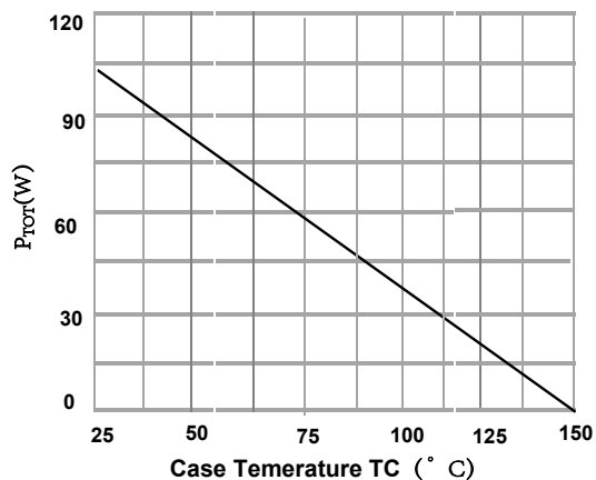
Fig. 12 P_{TOT} vs. T_C
