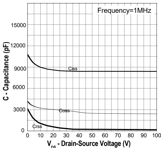
Fig11.Capacitance
